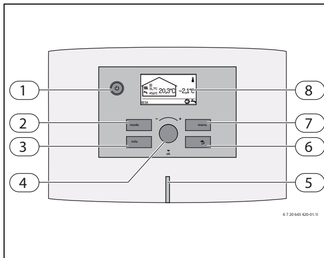
Joon. 3 Juhtpaneel
