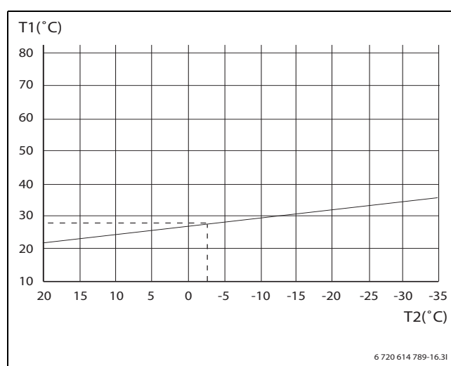
Joon. 22 Põrandaküte
