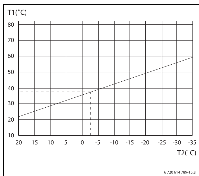
Joon. 21 Küttekeha
