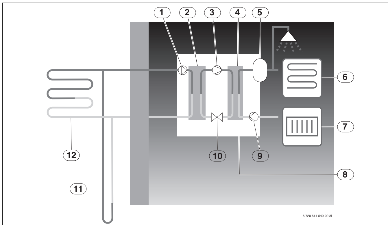
Joon. 2 Tööpõhimõte
